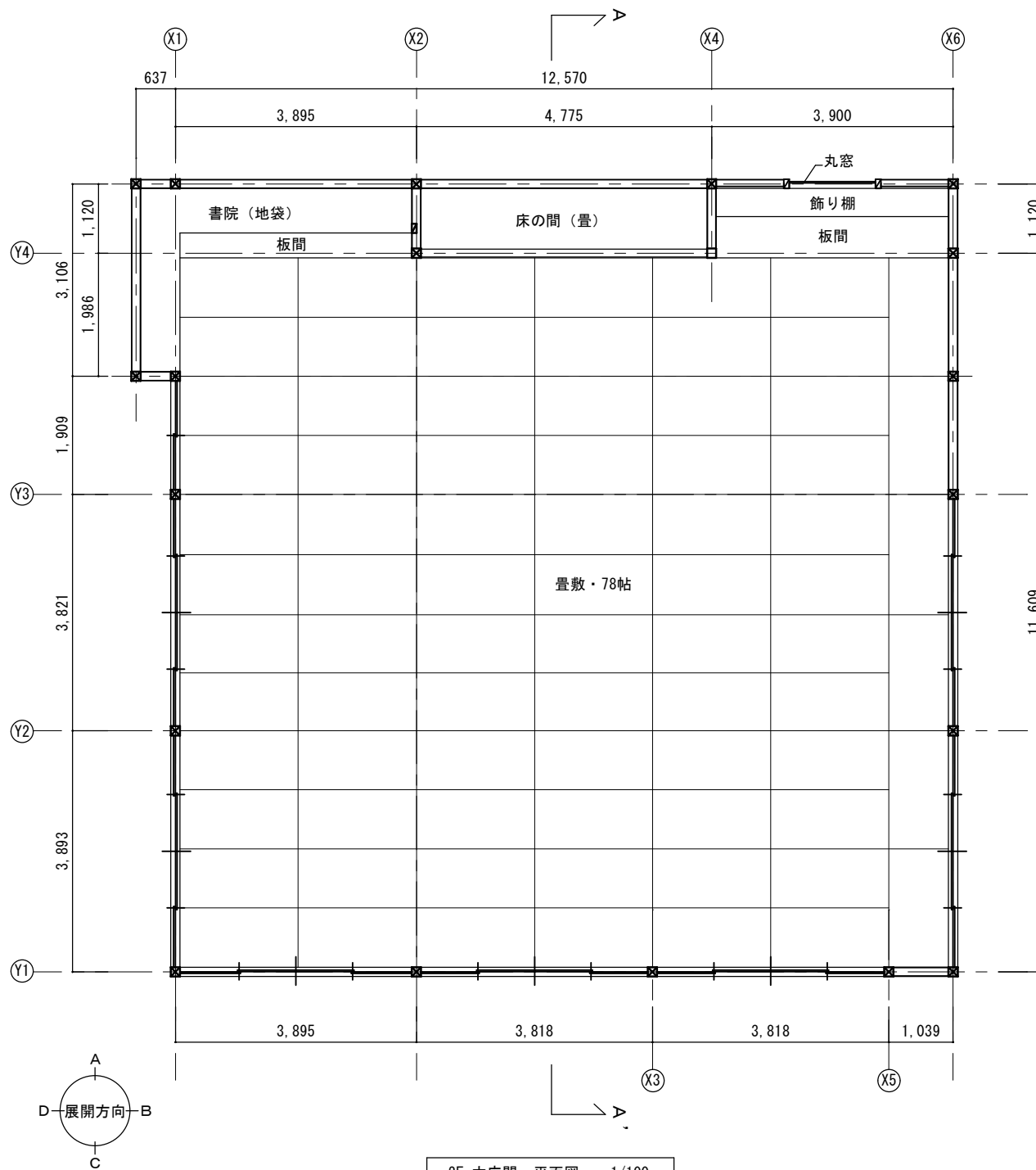
2F・大広間 平面図 1/100
